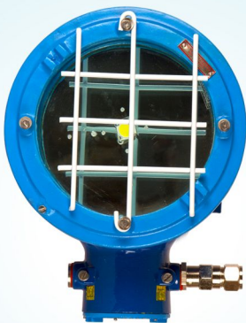
Exd.Bulkhead Luminaire
